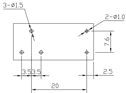
安装图
